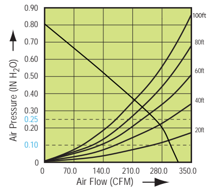
Pro300 Fan Curve
