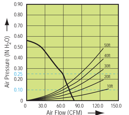
ITG70BT Fan Curve
