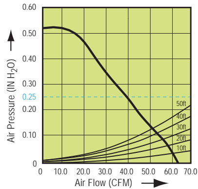
ITG50LED Fan Curve
