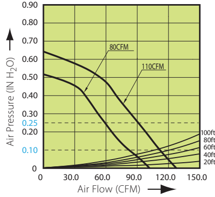
ELT80-110DLED / ELT80-110HLED ELT80-110MHLED Fan Curve
