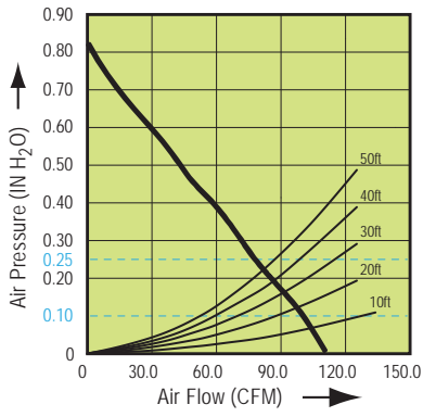
ITG100 Fan Curve
