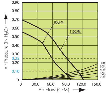
ELT80-110LED Fan Curve
