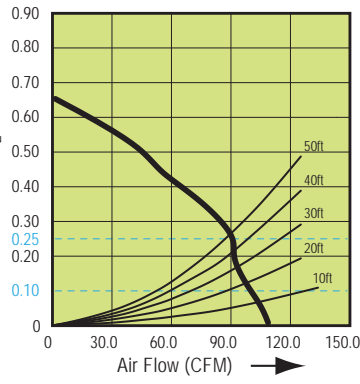
ITG100ELED Fan Curve
